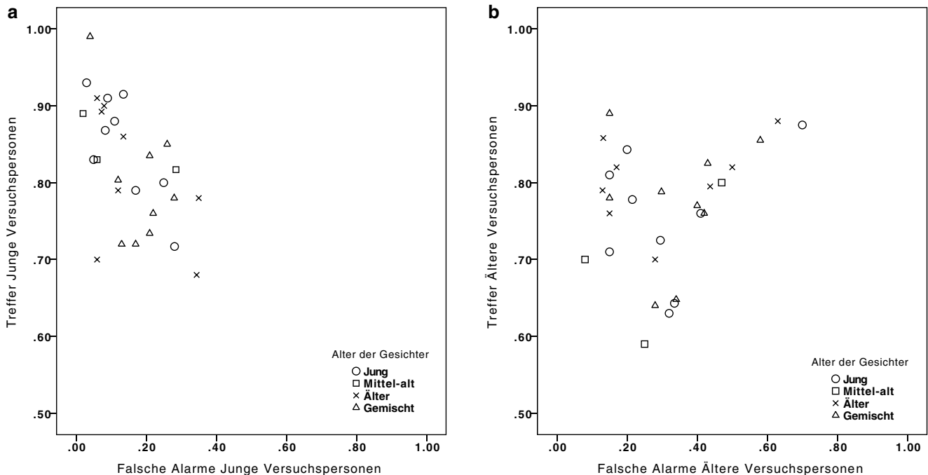
Abb. 2 Scatterplots des Zusammenhangs zwischen Treffern und falschen Alarmen für junge (a) und ältere Versuchsteilnehmer (b)
