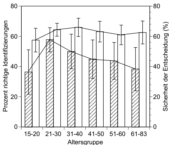
Abb. 3 Identifizierungsrichtigkeit (%) und subjektive Sicherheit (%) von Wählern verschiedener Altersgruppen. Schraffierte Balken Identifizierungsrichtigkeit, weiße Balken subjektive Sicherheit, Fehlerbalken 95 %-Konfidenzintervalle
