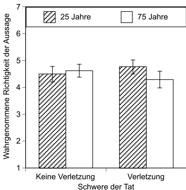
Abb. 4 Wahrgenommene Richtigkeit der Identifizierungsaussage (1 nicht zuverlässig, 7 sehr zuverlässig) in Abhängigkeit vom Alter des Opfers und der Schwere der Straftat (Fehlerbalken sind 95%-Konfidenzintervalle)
