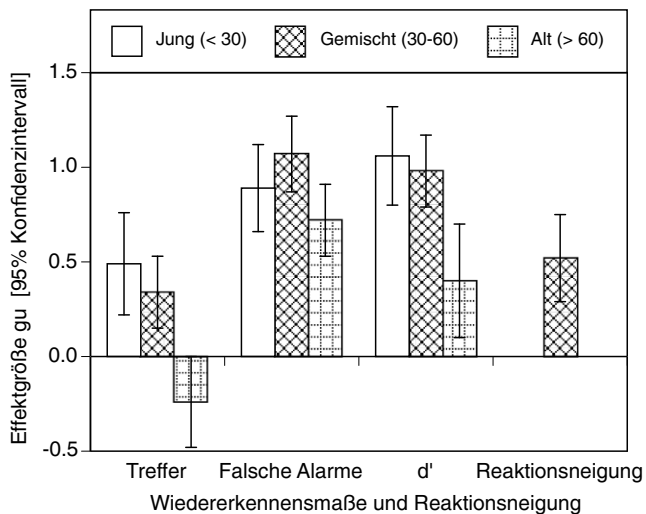
Abb. 1 Gewichtete mittlere Effektstärken für Treffer, falsche Alarme, Wiedererkennensleistung und Reaktionsneigung für Gesichter von jungen, Gesichter von jungen und älteren Personen gemischt und von älteren Personen
